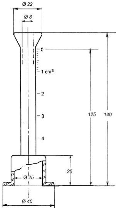
Рисунок 1. Трубка Карстена
